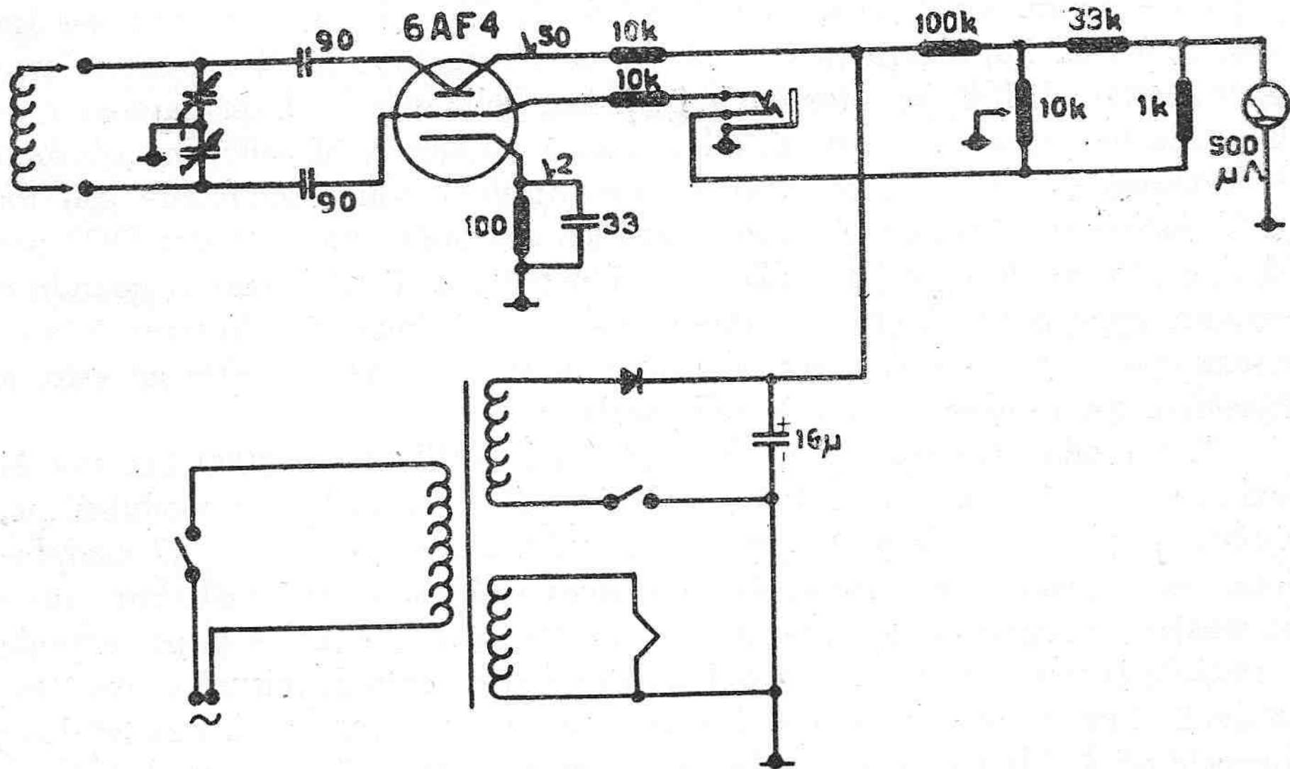
Fig. 92. - Ondametro ad assorbimento Heath GD-1 B.
