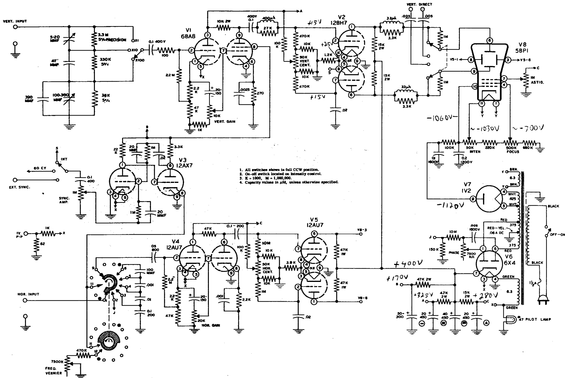
Fig. 2. Diagramme schématique de votre appareil.
