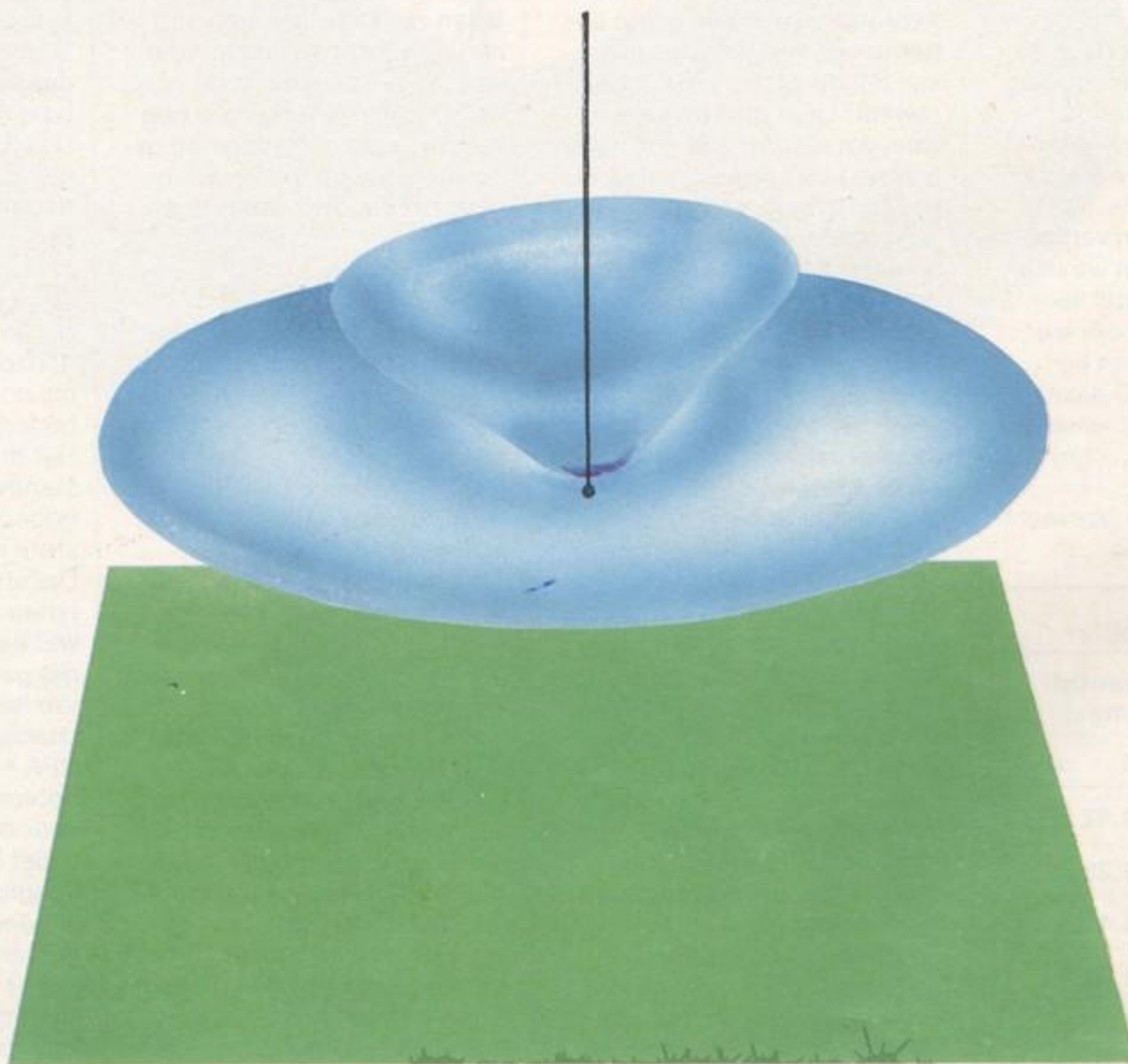
Fig. 13. 1/2 golf antenne op 2.75 m boven aarde.
