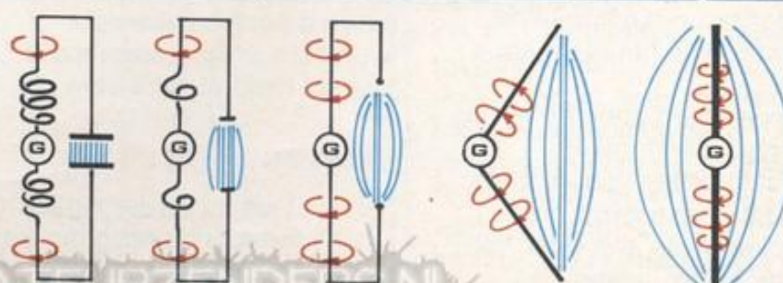
Fig. 2: Dipoolantenne gevormd uit spoel en condensator
