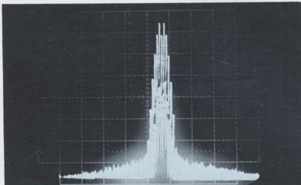
Nevenkanaal onderdrukking.
