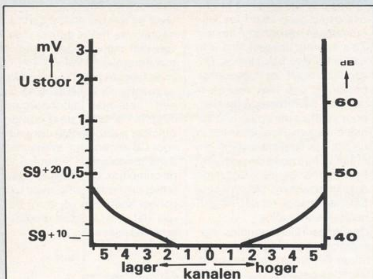
Fig. 9. Selectiviteit.
