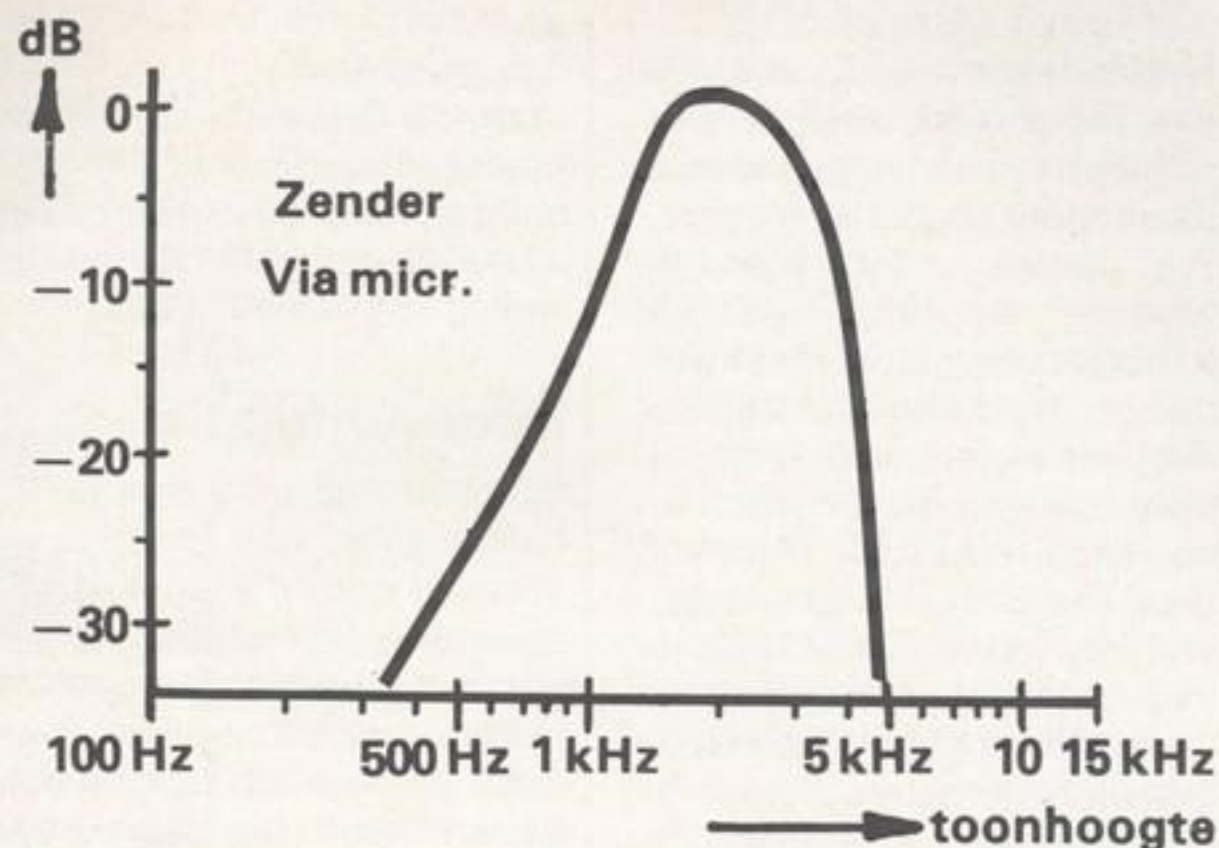
Fig. 4. Amplitude Frequentie karakteristiek.
