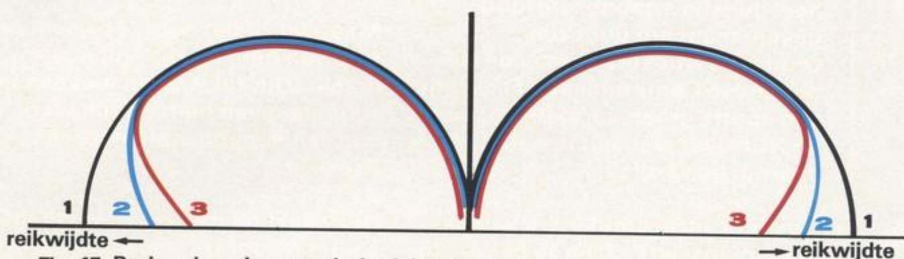
Fig. 15 Bodemdemping verminderd de reikwijdte
