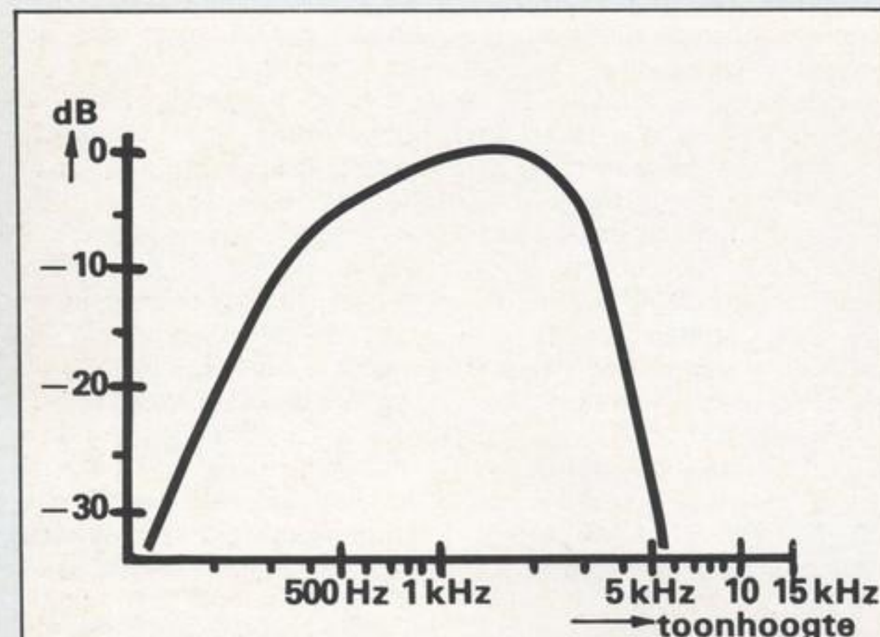
Fig. 9. Selectiviteit.
