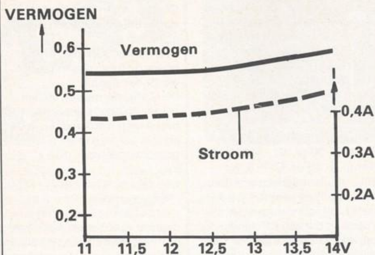
Fig. 1. Vermogen.
