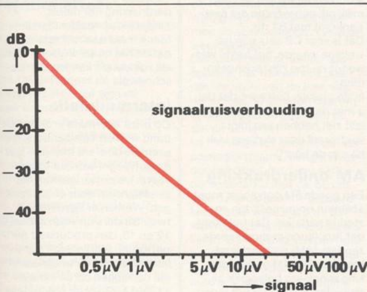
Fig. 6. Signaal/ruisverhouding.
