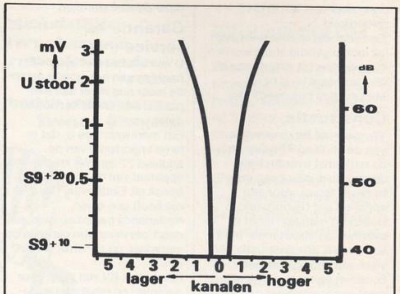
Fig. 9. Selectiviteit.
