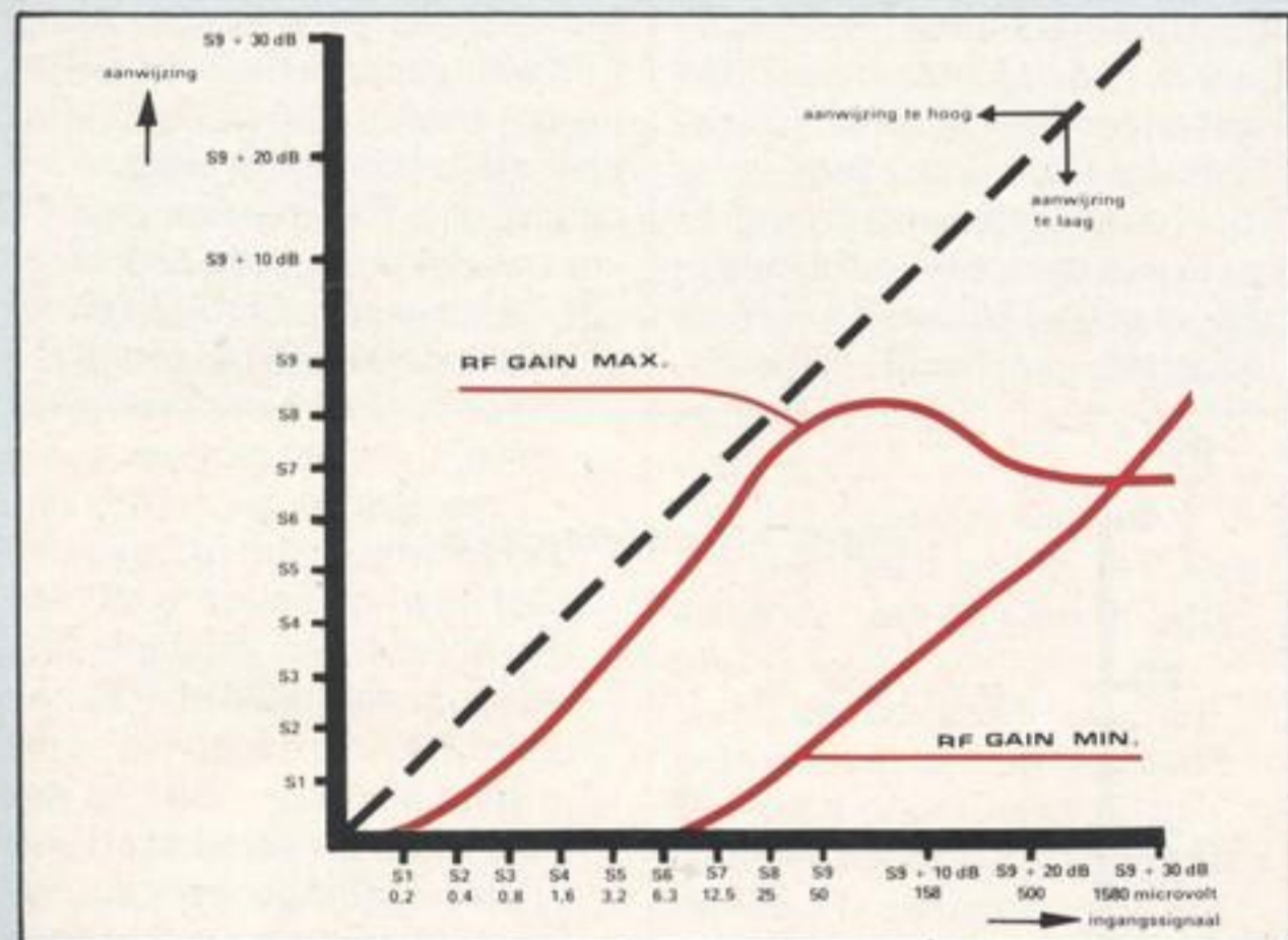
Fig. 6. Signaal/ruisverhouding.
