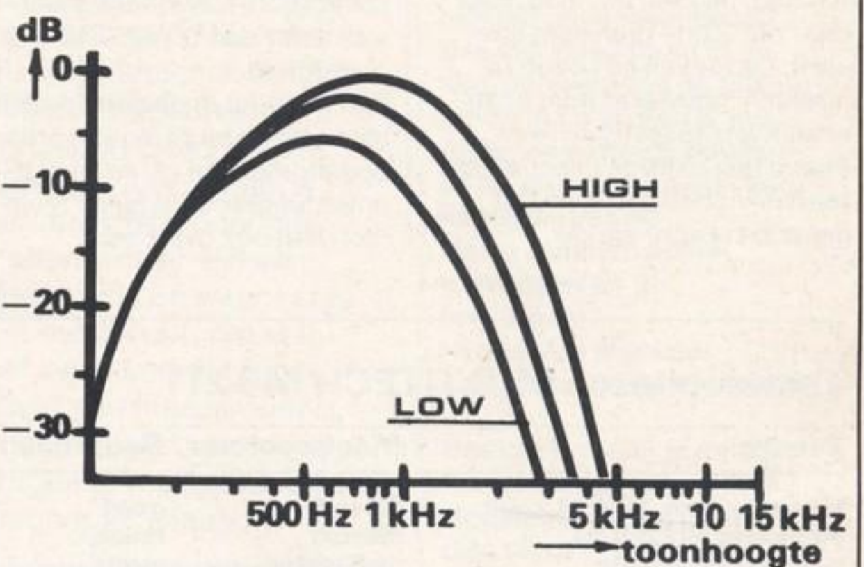
Fig. 10. Weergavebereik van de ontvanger.
