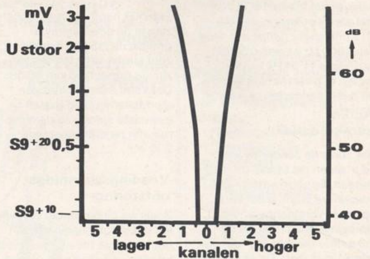
Fig. 9. Selectiviteit.
