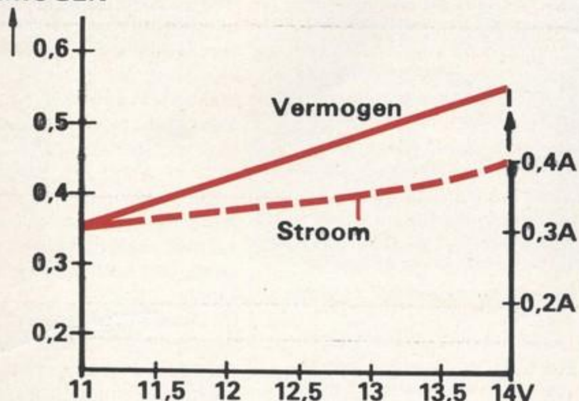
Fig. 1. Vermogen.
