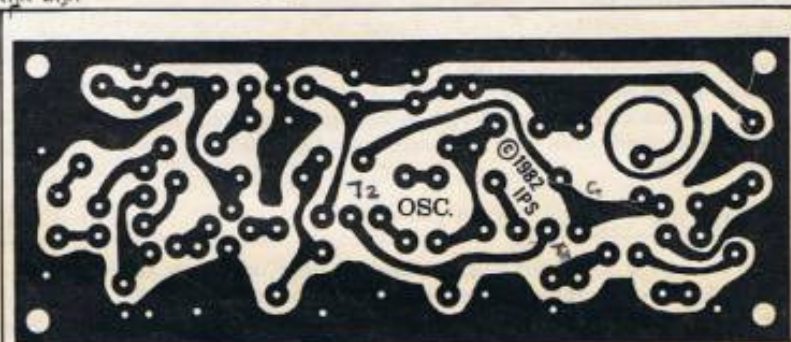
Koperzijde van de printlay-out (vare grootte).
