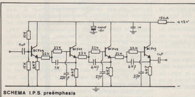
SCHEMA I.P.S. preëmphasis
