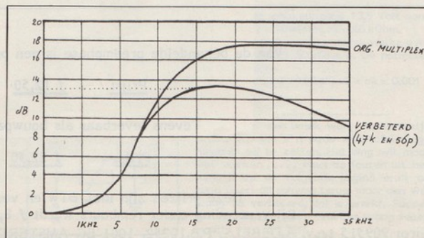
Verbeterd schema Multiplex FRM 4-'82
