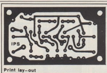
Print lay-out
