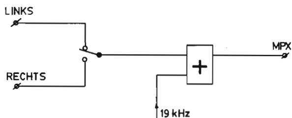
Fig.1 PRINCIPESHEMA STEREOCODER
