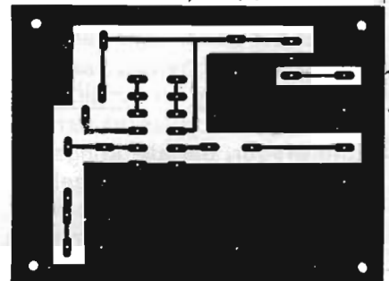
AF-ingang
