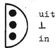
78L09, bovenzijde
