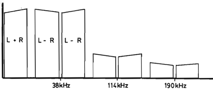
Fig. 4 FREQUENTIESPECTRUM MPX-SIGNAAL
