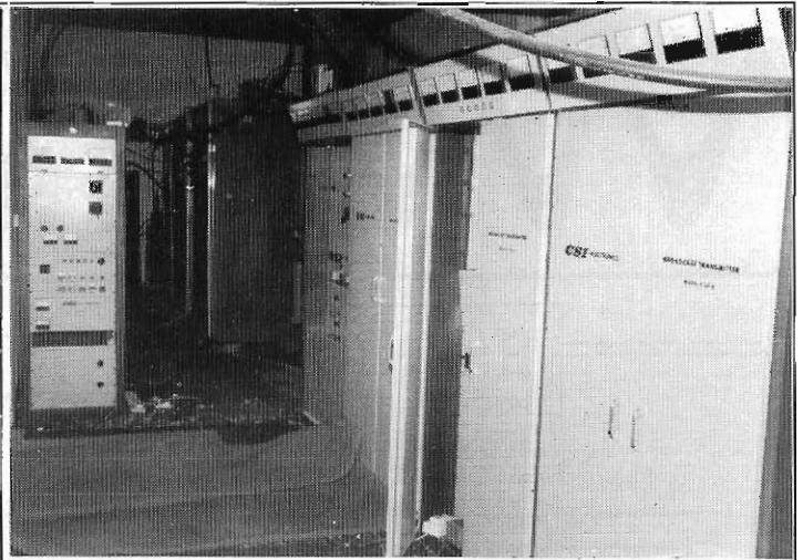
10 kW AM CSI/1 kW AM CSI/ 3 kW FM CSI en 50 kW AM RCA zenders. Links nog een 1 kW FM CSI zender.
