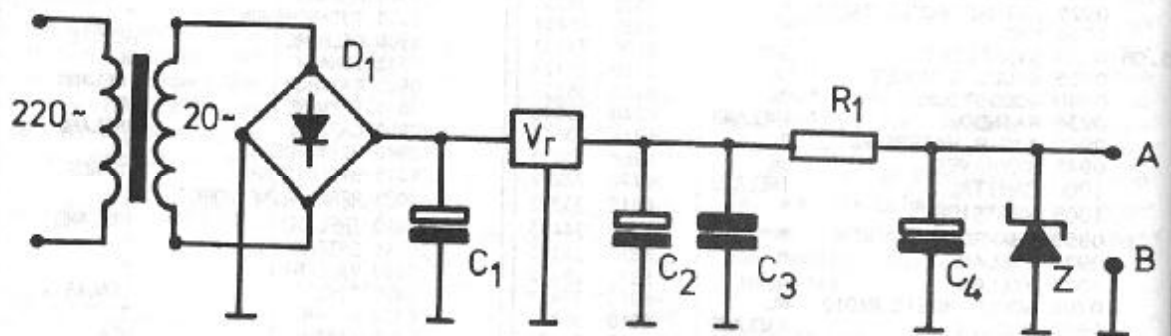
fig. 2 Voeding met resonantie-detector
