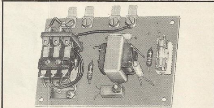
Fig. 4 - Aspetto della basetta a circuito stampato a montaggio ultimato.
