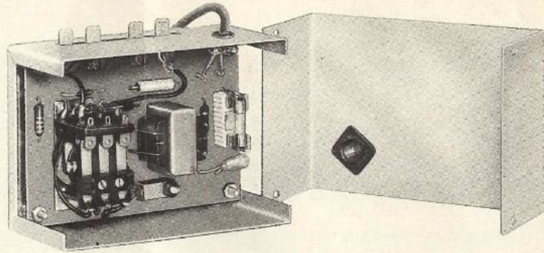
Fig. 6 - Disposizione dei componenti all'interno del contenitore.
