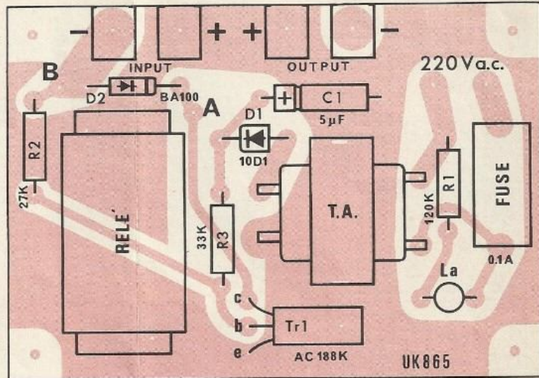
Fig. 2 - Serigrafia del circuito stampato.
