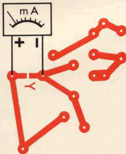
Fig. 3 - Connessione dei terminali del milliamperometro.
