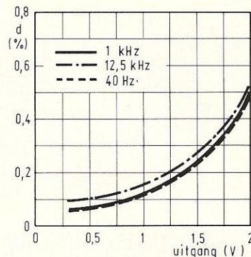
Afb. 3. Vervormingsfactor d van de mengversterker met een signaal op één ingang en kortsluiting van de andere ingang.
