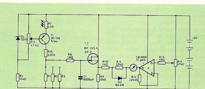
Afb. 4. Schema belichtingssterktemeter
