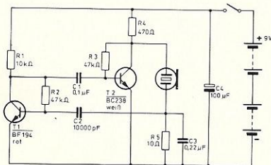
Afb. 6. Schema ultrasoontijdschakelaar a. zender
