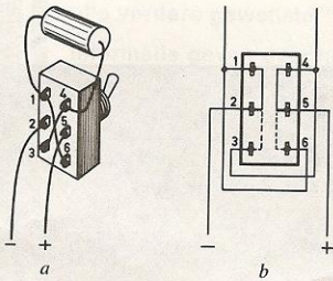
Afb. 13: Gebruikelijk type dubbele omschakelaar. In één stand wordt 1 en 2 verbonden en 4 met 5; in de andere stand 2 met 3 en 5 met 6. Vergelijk de stroomloop met afbeelding 12.
