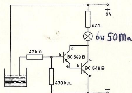
Afb. 5 Dit is een eenvoudige niveaumeter voor vloeistoffen die de elektriciteit enigszins geleiden, zoals gewoon water. Als de twee voelers, die van geleidend materiaal moeten worden gemaakt, door middel van de vloeistof worden „verbonden“, gaat het lampje branden.
