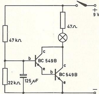
Afb. 3 Deze schakeling heeft een ingebouwde vertraging. Na het sluiten van de schakelaar duurt het enige tijd voordat de condensator is opgeladen en het lampje gaat branden. Bij gebruik van een terugverende drukknop moet de knop bewust een tijdje worden ingedrukt; even, per ongeluk, de knop indrukken heeft geen effect.
