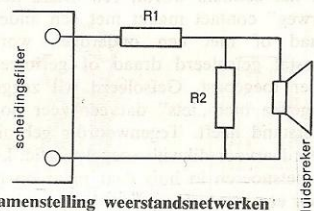
Samenstelling weerstandsnetwerken
