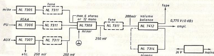
Voorbeeld van een combinatie van mengversterker-eenheden.
