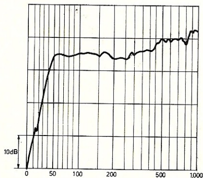
Frequentiekaracteristiek van de „Bombardon“ (AD 1255/W8)
