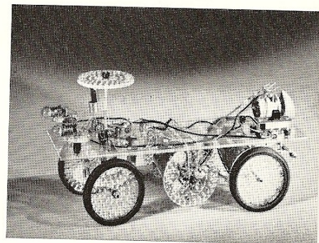
Een elektrowagen die reageert op licht en donker: combinatie van ME- en EE-onderdelen. Als de duisternis valt, remt de wagen af en ontsteekt de verlichting.
