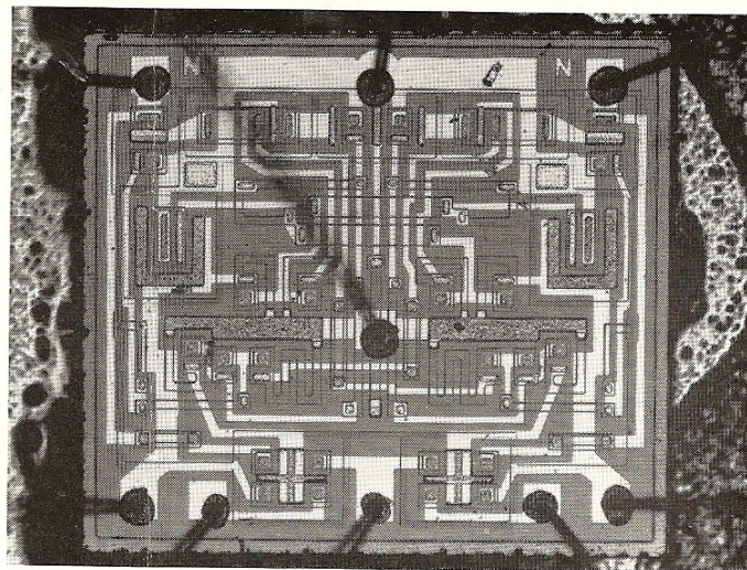
Elektronische microscheming met 51 onderdelen op 1,5 \times 1,3 mm.
