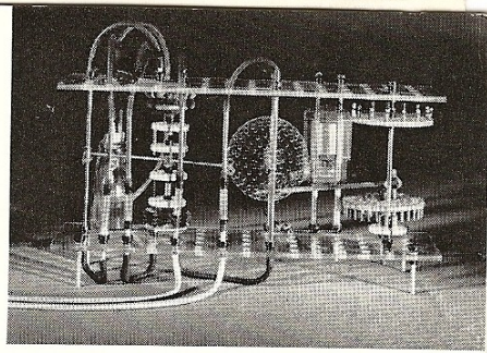
Dubbelwerkende waterpomp met twee in tegenfase werkende membraankamers.
