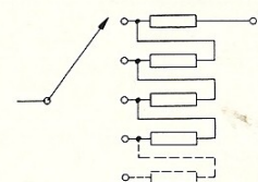
Afb. 2 Deze stappenschakelaar met vaste weerstanden kan in de plaats komen van R 7, R 8, R 9 en S 1. Voor het berekenen van de vaste weerstanden: zie tekst.
