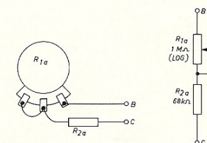
Afb. 3a Regeling van de snelheid met een logaritmische potentiometer (linksom sneller).
