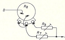
Afb. 1a Detail voor aansluiting potentiometer R 8.
