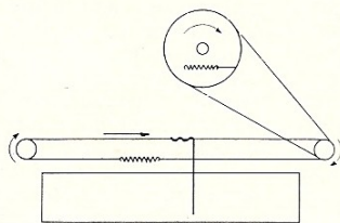
Afb. 1 Bij deze afsteminrichting kan het spanveertje zowel in de trommel als in de snaar zelf worden aangebracht. De snaar bestaat uit één stuk.
