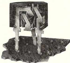
Opengewerkt model van een „lock-fit“-transistor
