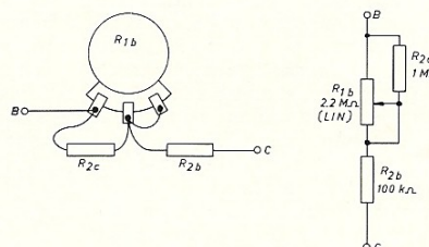
Afb. 3b Regeling met een lineaire potentiometer (rechtsom sneller).
